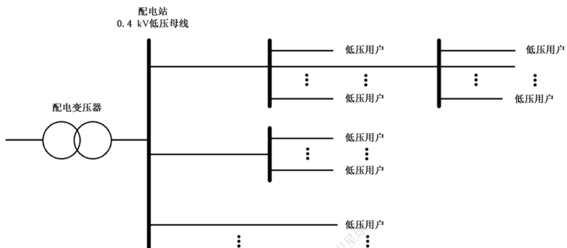
图 C.1 辐射式
